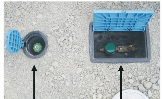
不凍栓(左)とメーターボックス(右)
