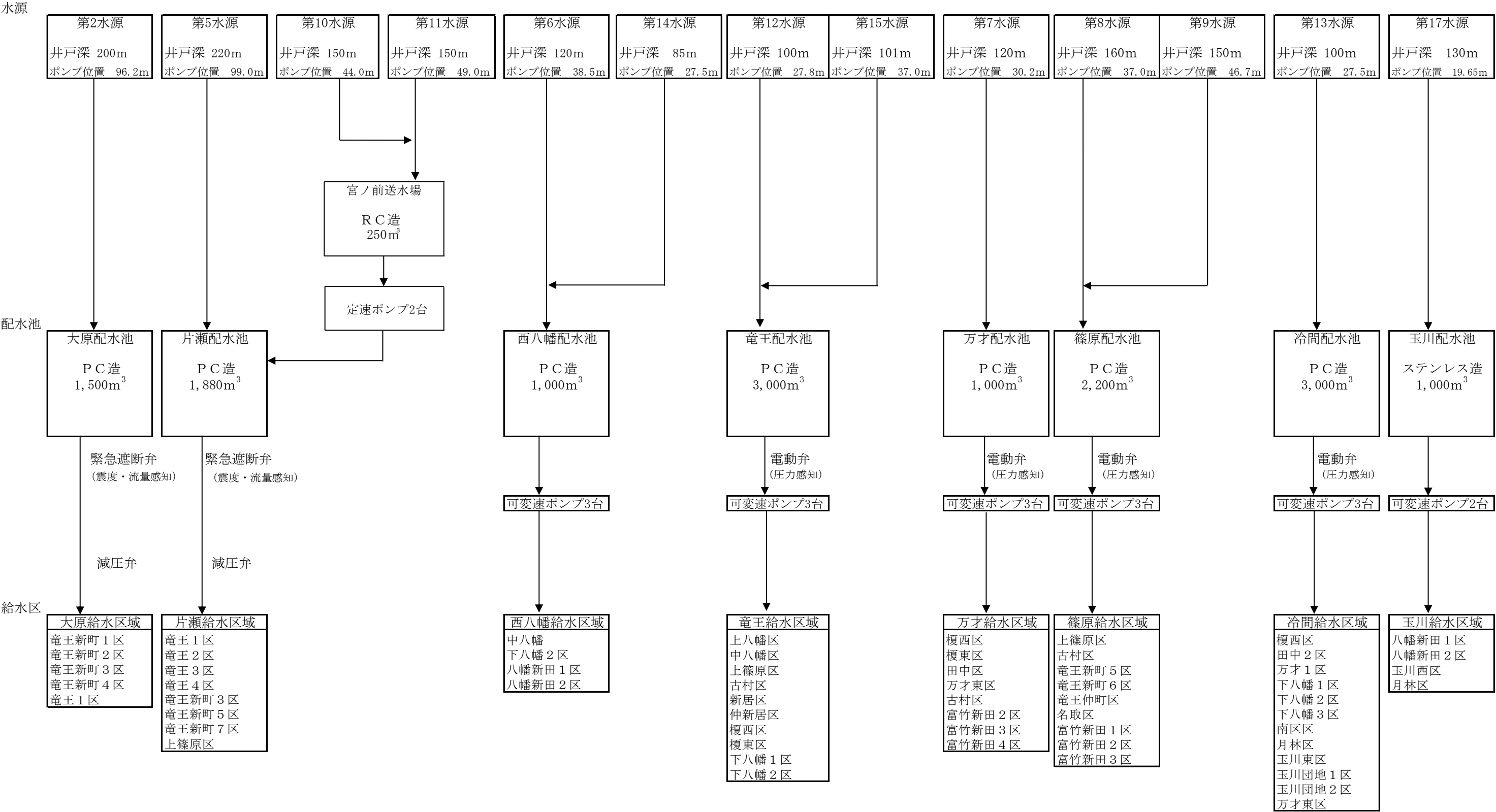
甲斐市竜王地区配水系統図
