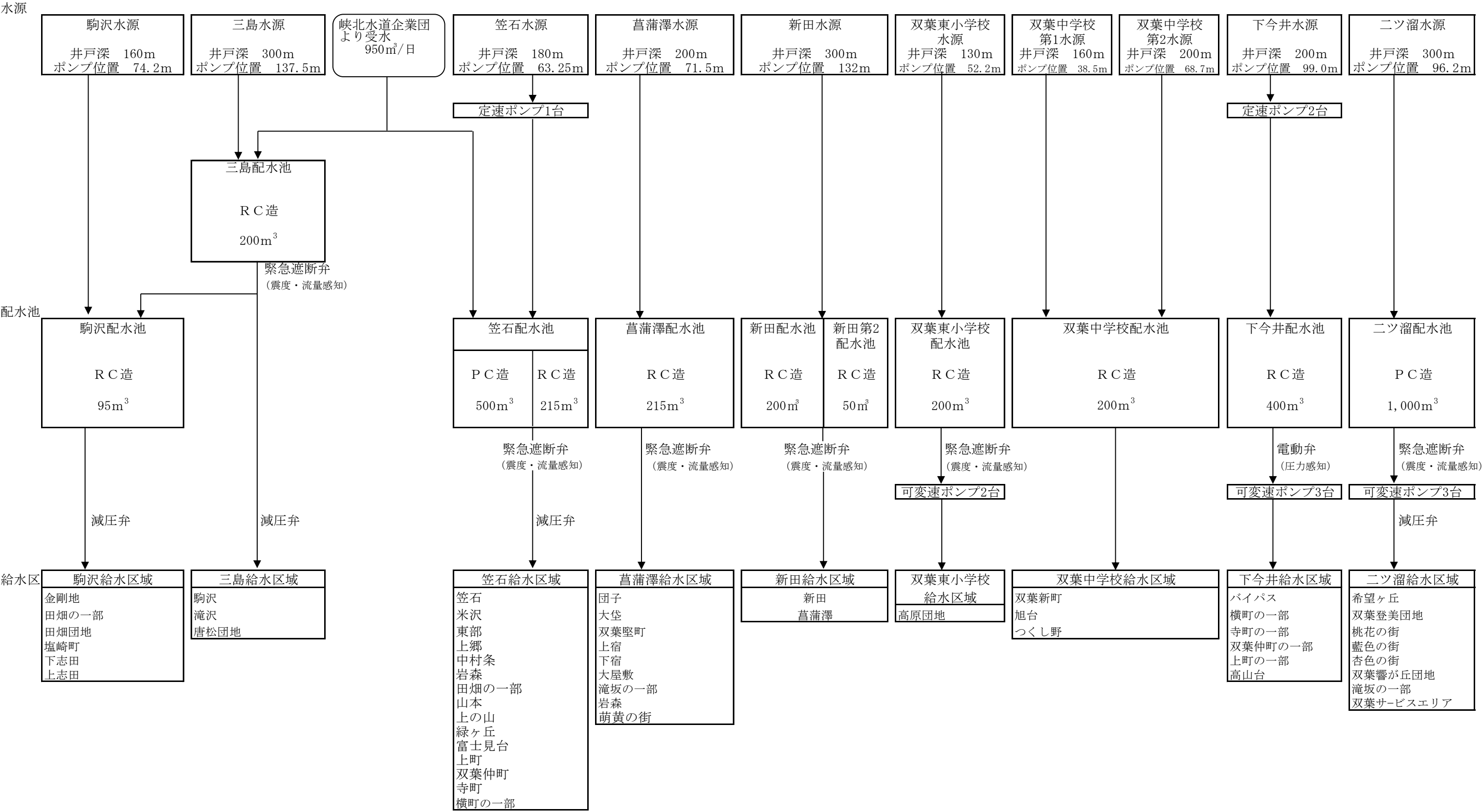
甲斐市双葉地区配水系統図
