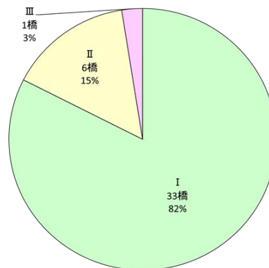
図-2 健全性の診断結果
